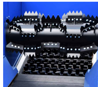
Dosing Rotor
